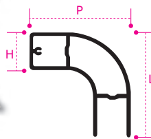
Complete Corner Profile with Caps Angolare Completo di Tappi
