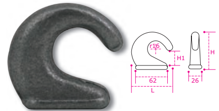
Light Towing Hook Gancio Traino Leggero
